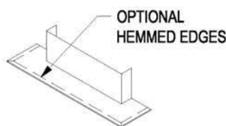
APRON FLASHING
